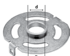
KR-D 24,0/OF 1400 für OF 1400 / VS 600; passend für die Schablonen SZ 20 und SZO 20 des Verbindungssystems VS 600; selbstzentrierend; werkzeuglos einsetzbar
