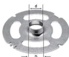
KR-D 24,0/OF 2200 für OF 2200; geeignet für Fräser bis 19 mm Durchmesser
