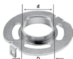
KR-D 40,0/OF 1400 für OF 1400; geeignet für Fräser bis 35 mm Durchmesser
