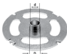
KR-D 17,0/OF 2200 für OF 2200; geeignet für Fräser bis 12 mm Durchmesser
