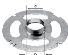
KR-D 30,0/OF 2200 für OF 2200; geeignet für Fräser bis 25 mm Durchmesser
