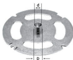
KR-D 12,7/OF 2200 für OF 2200; Kopiererring in Zoll-Größe
