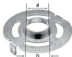
KR-D 30,0/OF 1400 für OF 1400; geeignet für Fräser bis 25 mm Durchmesser
