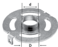
KR-D 27,0/OF 1400 für OF 1400; geeignet für Fräser bis 22 mm Durchmesser
