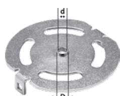
KR-D 8,5/OF 1400 für OF 1400 / VS 600; passend für die Schablone SZO 14 Z des VS 600 Verbindungssystems; passend für die Schablone FZ 6 des VS 600 Verbindungssystems; selbstzentrierend; werkzeuglos einsetzbar
