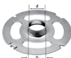
KR-D 27,0/OF 2200 für OF 2200; geeignet für Fräser bis 22 mm Durchmesser
