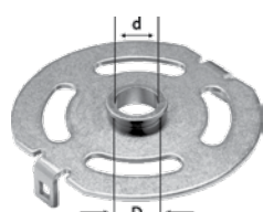
KR-D 17,0/OF 1400 für OF 1400 / VS 600; passend für die Schablonen SZ 14 und SZO 14 des Verbindungssystems VS 600; selbstzentrierend; werkzeuglos einsetzbar
