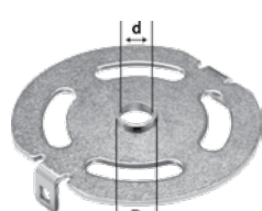
KR-D 13,8/OF 1400 für OF 1400 / VS 600; passend für die Schablone SZO 20 des VS 600 Verbindungssystems; passend für die Schablone FZ 10 des VS 600 Verbindungssystems; passend für die Schablone DS 32 des VS 600 Verbindungssystems; selbstzentrierend; werkzeuglos einsetzbar
